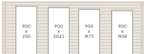
Door dimensions
